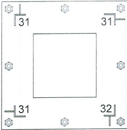
Section A-A PL80*80*0.8
