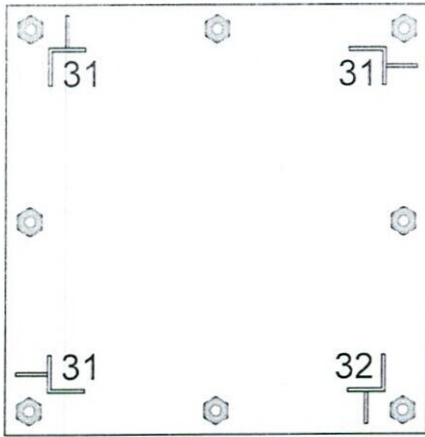
Section A-A PL800*800*12
