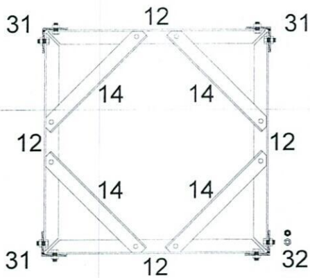
Section C-C & D-D
